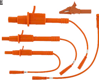
PRÜFKABELSATZ FÜR ELEKTRO- / HYBRID- FAHRZEUGE
