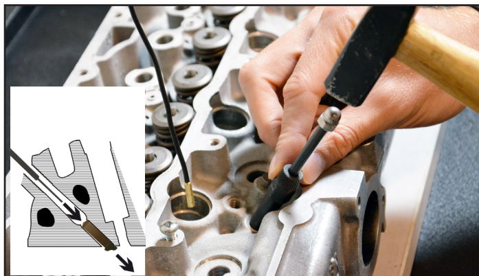
CHASSE POUR CRAYONS ÉVASÉS ET BLOQUÉS DOORSLAG VOOR GEBLOKKEERDE STIFTEN
